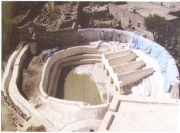
سور فناء بركة الوضوء وكتلة المدخل الغربي أثناء أعمال الترميم
